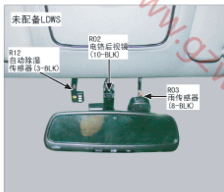
143. 前挡风玻璃
