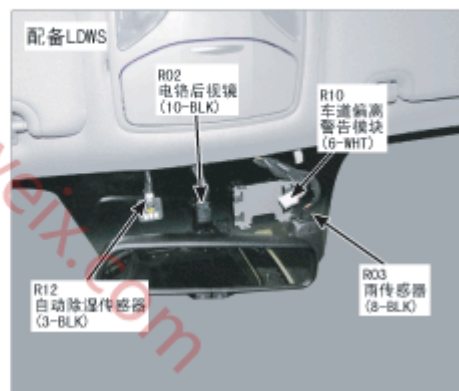
144. 前挡风玻璃
