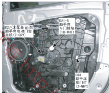
140. 助手席车门
