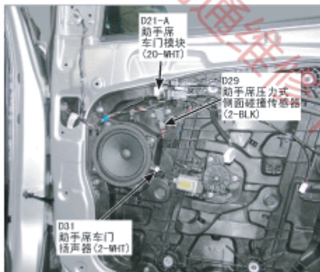
139. 助手席车门
