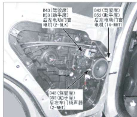
141. 后车门
