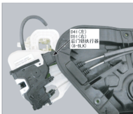
142. 后车门模块
